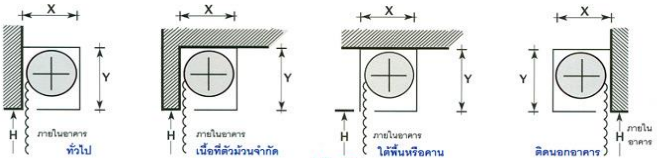
รูปตัด (A)
