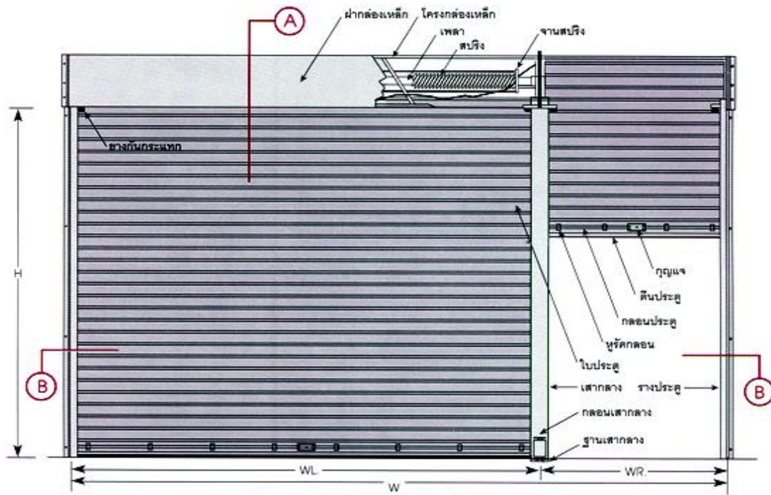
รูปด้านแสดงรายละเอียดและอุปกรณ์ประตูม้วน
